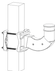
Poste Cuadrado Vertical
