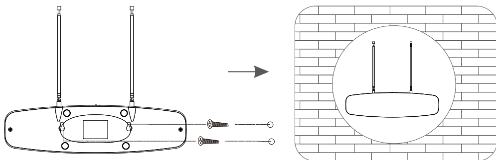
Montaje horizontal
